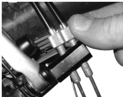
Obr. 139: Náboje Rohloff s vnitřním ovládáním řazení mají nastavovače napnutí na držáku protitahu
