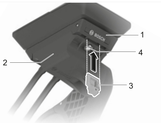
Obr. 108: Umístění šroubu hlavního složení
