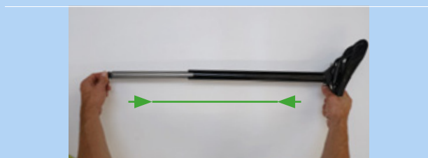
Obr. 202: Stlačení sedlovky
