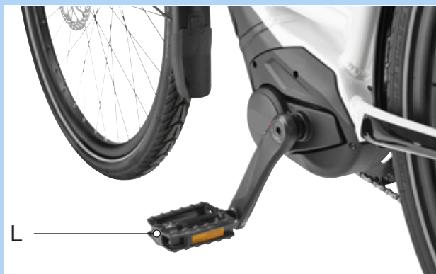
Obr. 85: Pedál L levého ramena kliky
