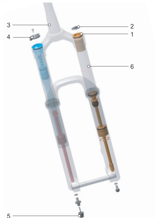
Obr. 15: Vnitřní konstrukce vidlice se vzduchovým pružením
