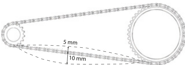
Obr. 166: Příklad kontroly napnutí řetězu: 5 mm dolů, 10 mm nahoru = výchylka 15 mm
