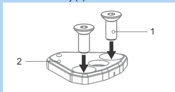
Obr. 81: Zasunutí šroubů se zápusťnou hlavou do základové desky
