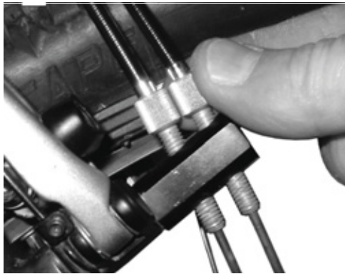
Obr. 189: Náboje ROHLOFF s vnitřním ovládáním řazení mají nastavovače napnutí na držáku protitahu
