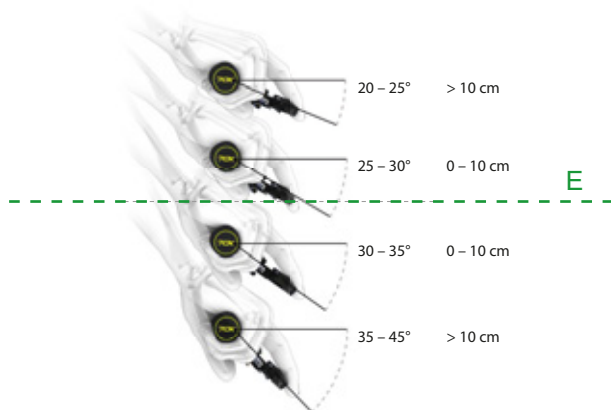
Obr. 120: Úhel sklonu brzdy
