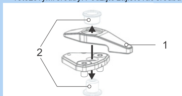
Obr. 82: Pojistnou páku spojte se základovou deskou
