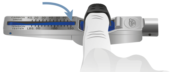
Obr. 180: Ukazováček v kontrolním měřidle
